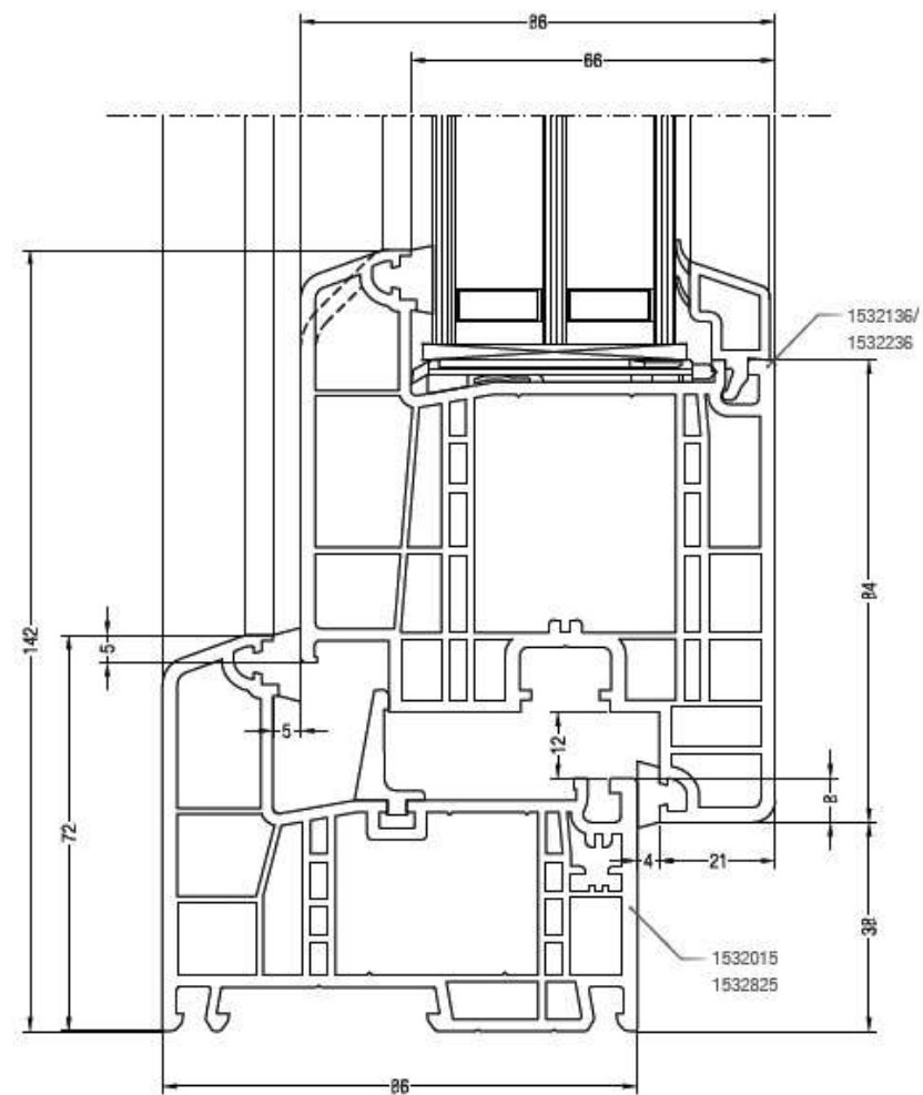
Sezione nodo anta dritta da 84 mm
