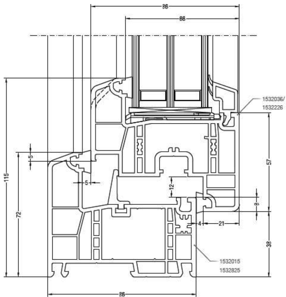
Sezione nodo anta dritta da 57 mm
